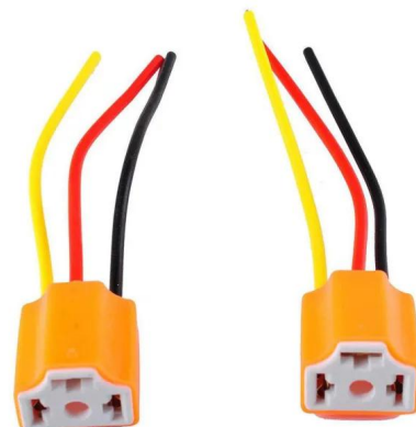
CONECTOR DE LÁMPARA FRONTAL PARA H4 (RECTO) - CERÁMICO (10 PCS)
